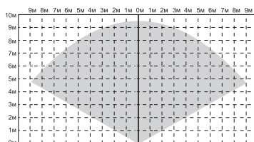
Схема зони охоплення датчика
