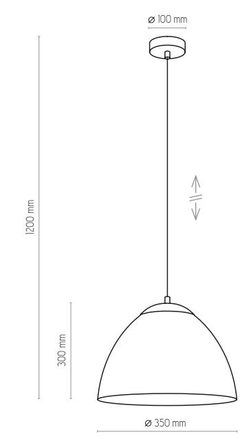
3193 | FARO | 1x E27, max 60W
