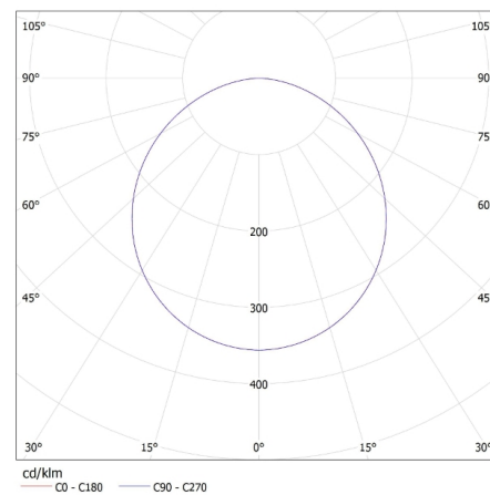
MILEDO (kat 31082) SP LED N 18W NW-S / LDC (Polar)
