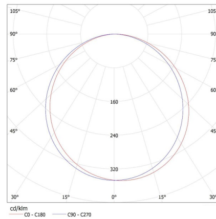
KANLUX S.A. (kat 28021) BRAVO P 36W12030NW SR / LDC (Polar)
