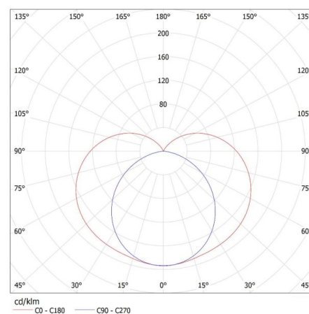
KANLUX S.A. (kat 27532) PESSA LED IP44 17W-WW / LDC (Polar)
