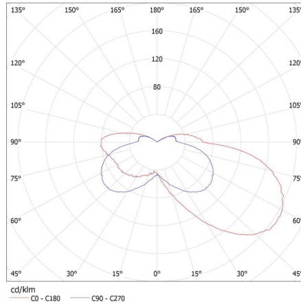
KANLUX S.A. (kat 27375) SABIK LED PIR CW / LDC (Polar)
