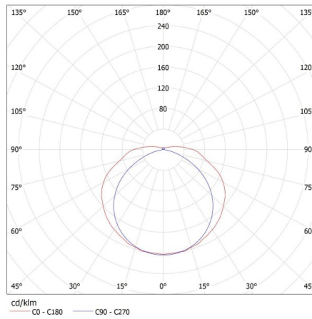
KANLUX S.A. (kat 26960) MEBA 4LED 2X60 PS + Miledo / LDC (Polar)
