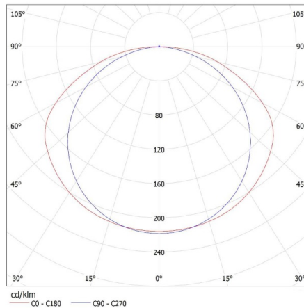
KANLUX S.A. (kat 26375) ALDO 4LED 2X150R + Miledo / Krzywa rozsyłu światła (biegunowo)
