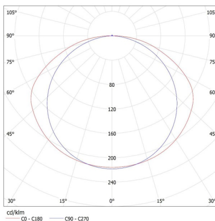
KANLUX S.A. (kat 26373) ALDO 4LED 2X60R + Miledo / Krzywa rozsyłu światła (biegunowo)
