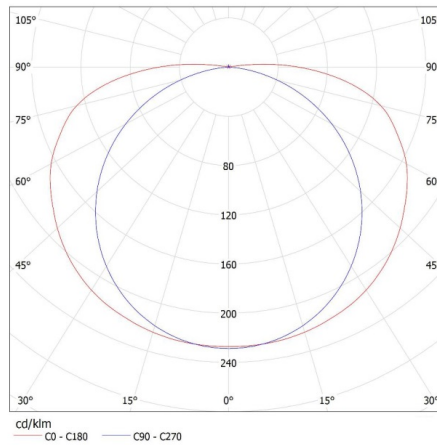
KANLUX S.A. (kat 26371) ALDO 4LED 1X120R + Miledo / Krzywa rozsyłu światła (biegunowo)
