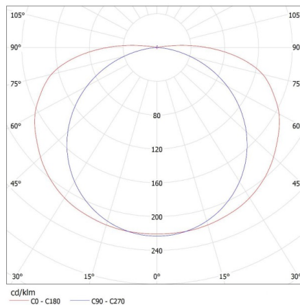
KANLUX S.A. (kat 26370) ALDO 4LED 1X60R + Miledo / Krzywa rozsyłu światła (biegunowo)
