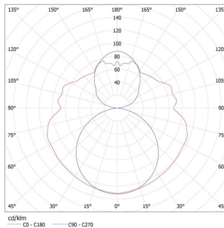
KANLUX S.A. (kat 26363) ALDO 4LED 2X60 + Miledo / Krzywa rozsyłu światła (biegunowo)
