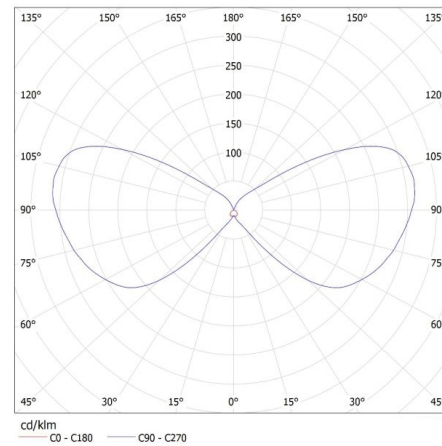
KANLUX S.A. (kat 23790) RUBINAS 2LED-WW / Krzywa rozsyłu światła (biegunowo)
