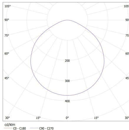
KANLUX S.A. (kat 23710) PIRMO LED SMD NW / Krzywa rozsyłu światła (biegunowo)
