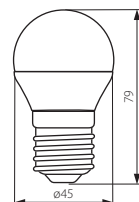
BILO 6,5W T SMD E27
