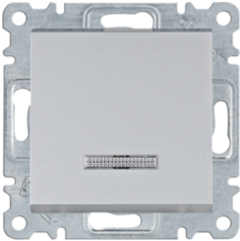
Вимикач з пі дсві чуванням 1-полюсний Lumina, срі бний, 10AX/230В
