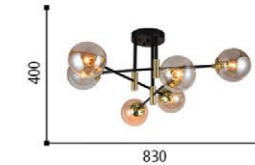
6718-46 ∅ 830 ↑↓ 400 ⚡ E27 220V 6 x 40W IP20 metal, glass
