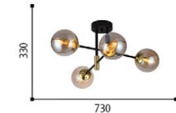
6718-44 ∅ 730 ↑↓ 330 ⚡ E27 220V 4 x 40W IP20 metal, glass
