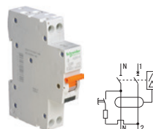
Дифференциальный автоматический выключатель АД63 К
